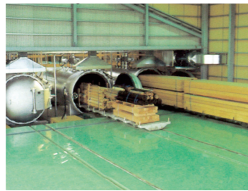
加圧注入による防腐処理
